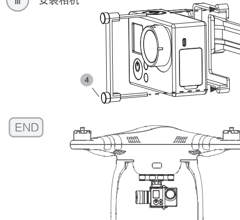
V型挂架
