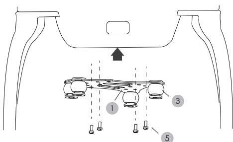
上挂板
